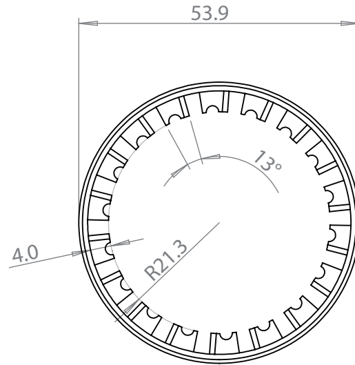
inner lid
