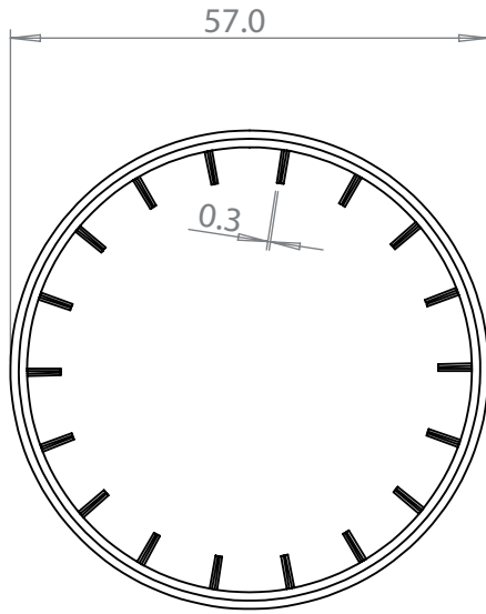
out lid
