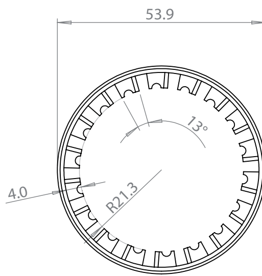
inner lid
