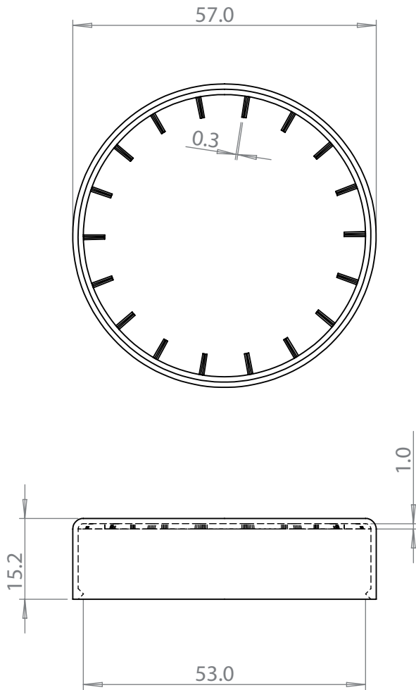
out lid
